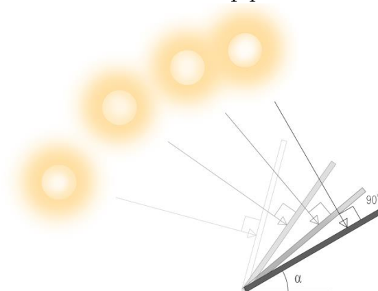
Рисунок 6. Зависимость угла наклона \alpha солнечной панели от широты местности
